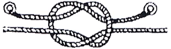
Nodo piatto
