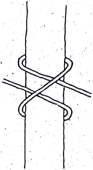
Nodo barcaiolo
